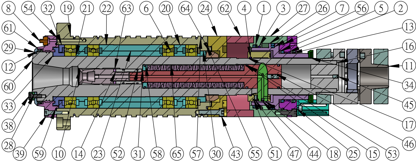
剖面圖 A-A
